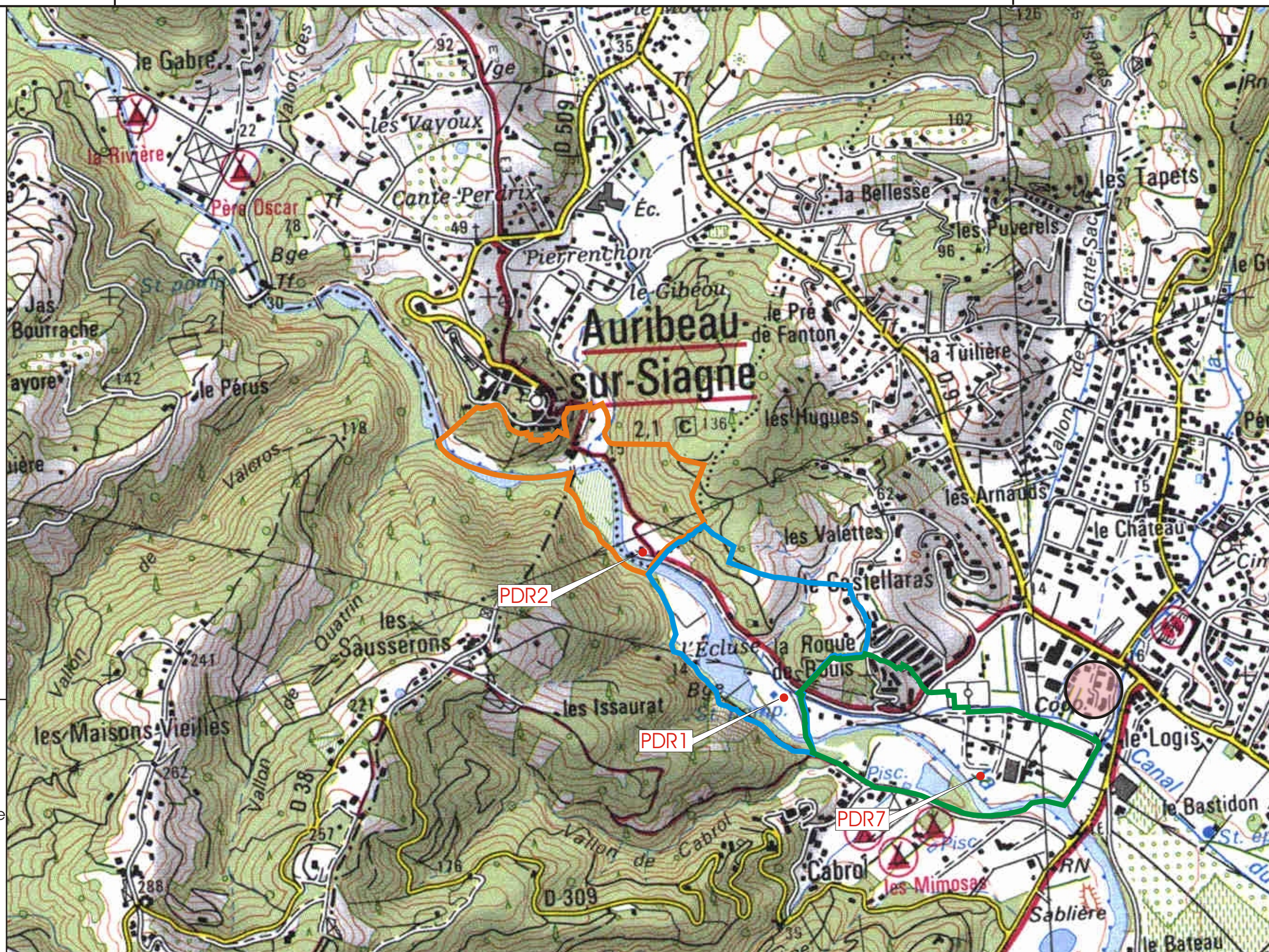
Figure 10 PERIMETRES DE PROTECTION RAPPROCHEE SUR PLAN TOPOGRAPHIQUE
